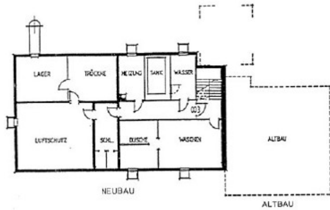
UNTERGESCHOSS
